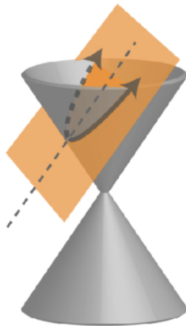
Parabola
