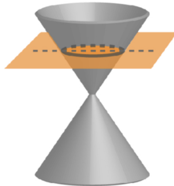
Circle
